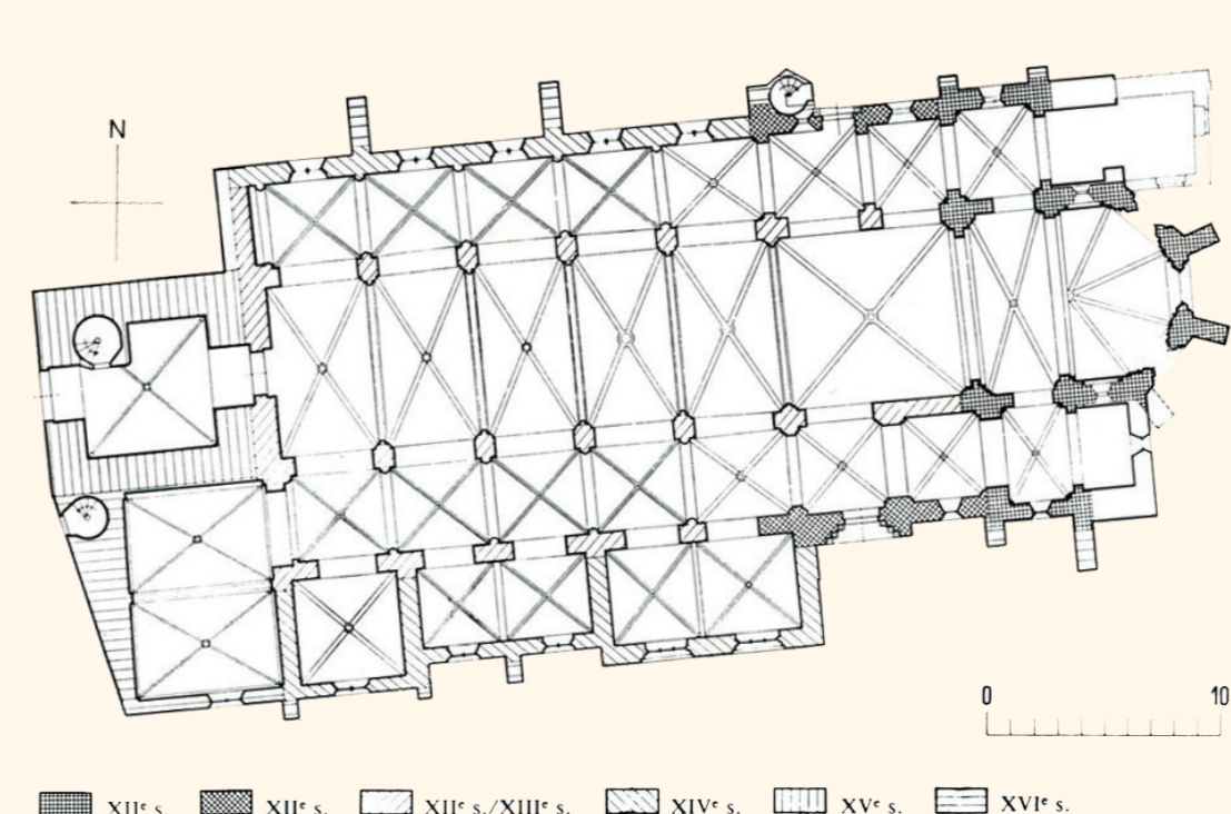
Plan de la Collégiale, avant la restauration de 1964
