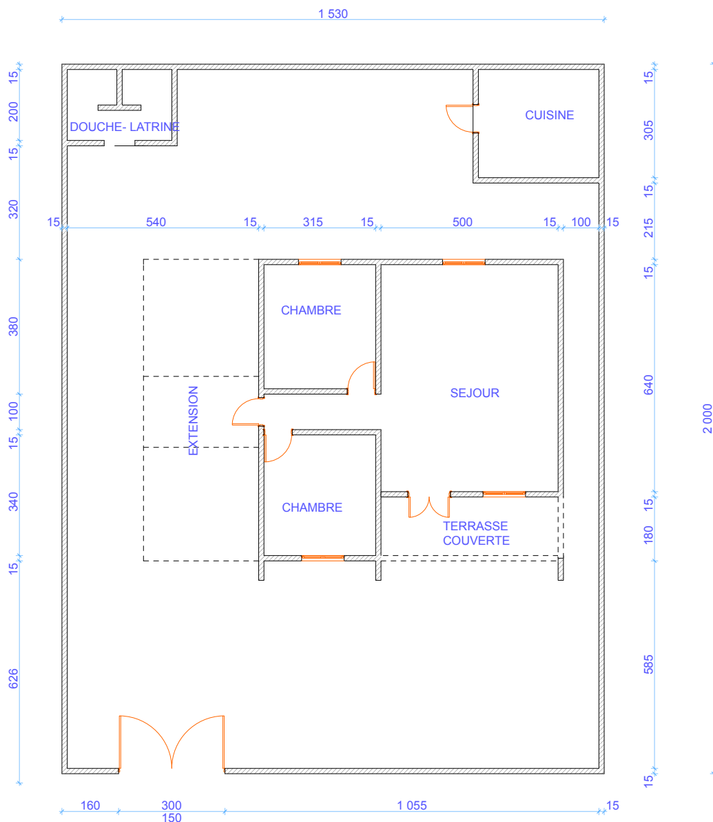
PLAN DE LOGEMENT F3 INITIAL
