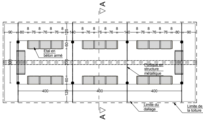
PLAN DE NIVEAU D'UN MODULE DE HANGAR (22 places)
